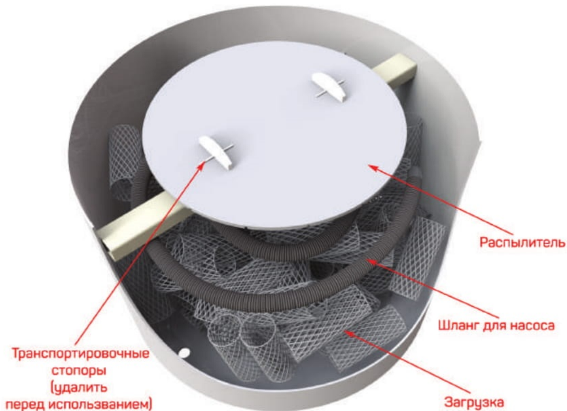
Рис. 1 - Корзина с загрузкой
