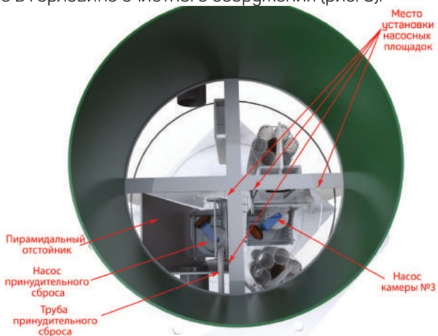
Рис. 3 – Станция, вид сверху
