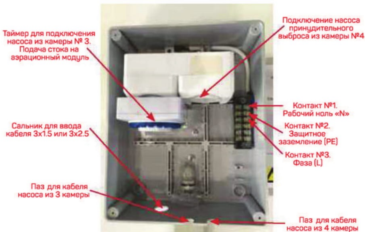
Рис. 5 – Подключение блока управления
